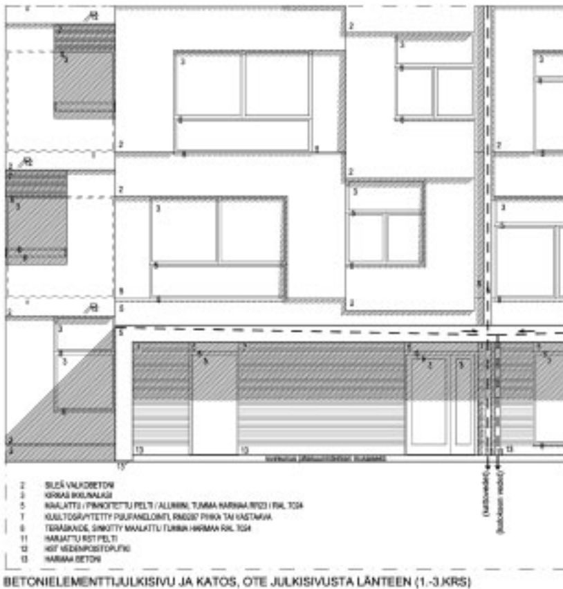
BETONIELEMENTTIJULKISIVU JA KATOS, OTE JULKISIVUSTA LÄNTIEN (1.-3.KRS)
