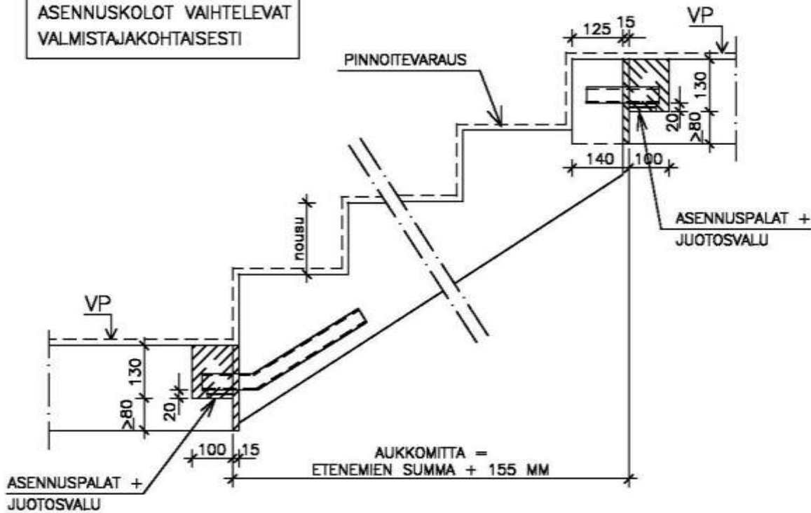
Kuva 5 Sivupalkiton umpilaattaporras
