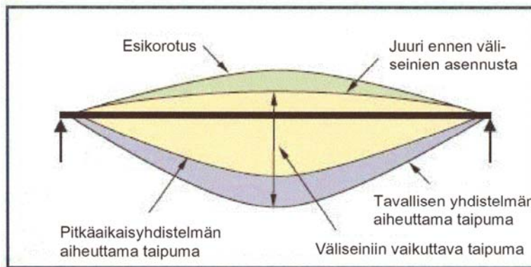
Kuva 7. Laatan esikorotus
