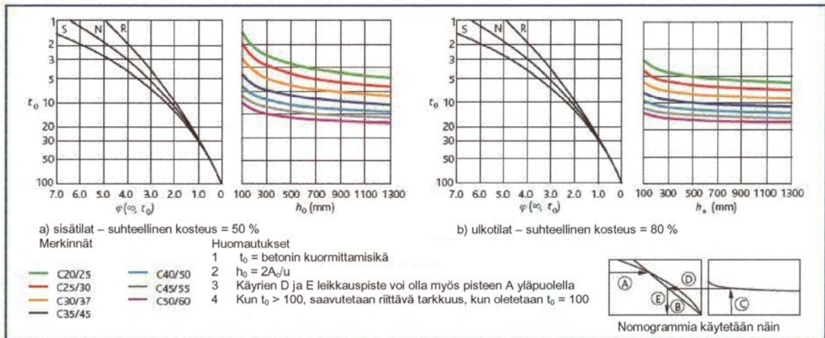
Kuva 5 Virumaluvun \varphi(\infty, t_0) määrittäminen
