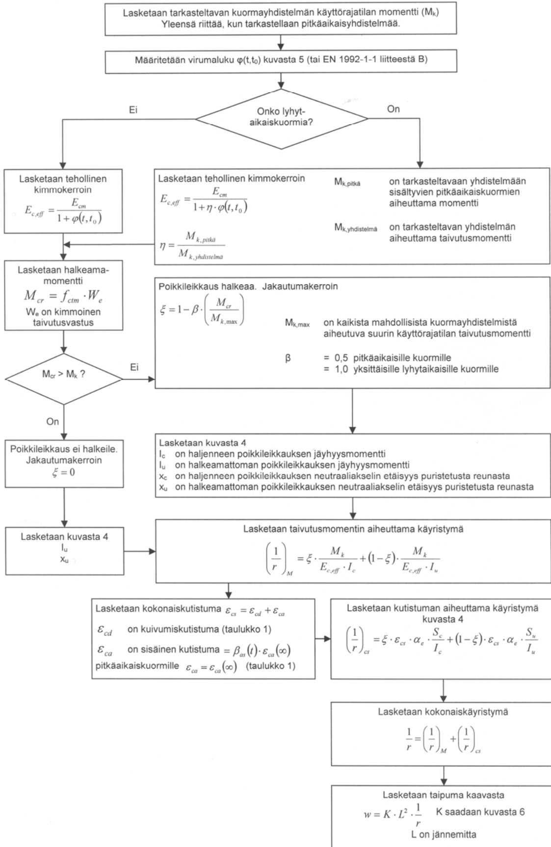
Kuva 3. Taipuman laskenta
