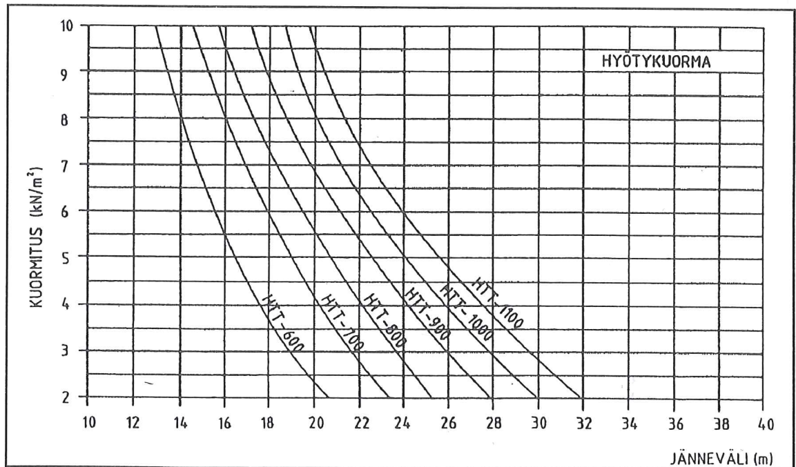
Kuva 7.47 HTT-laatan kantokyky, kaltevuus 1:40, normaalibetoni
