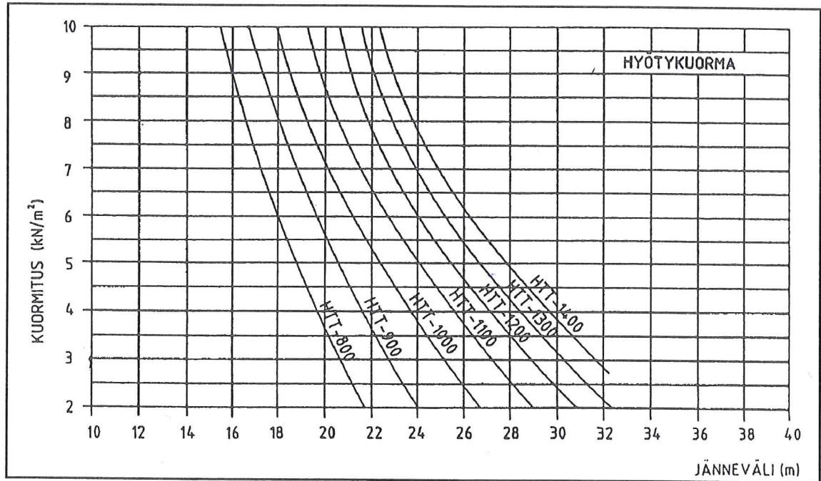
Kuva 7.46 HTT-laatan kantokyky, kaltevuus 1:20, normaalibetoni
