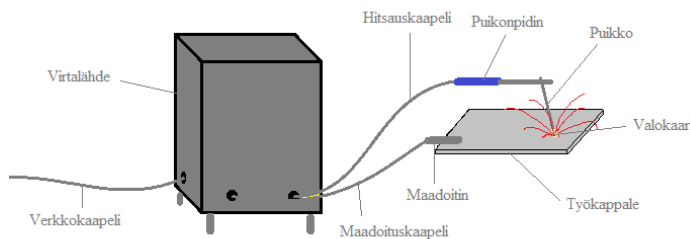
Kuva 7. Puikkohitsauslaitteen komponentit [15].
