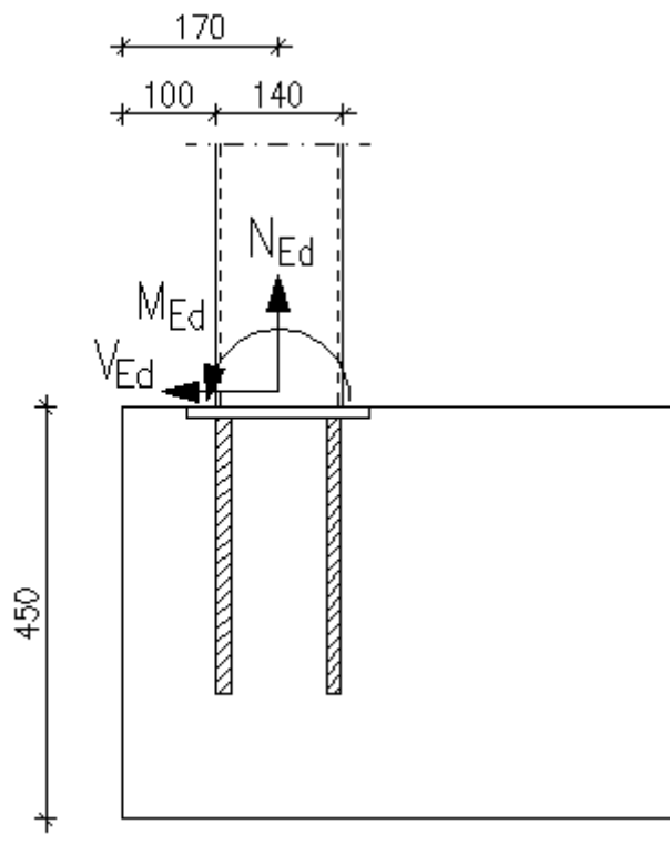
Kuva 4. SBKL-kiinnityslevyn mitoitusesimerkki ilman lisäraudoitusta, kiinnityslevyn rakennemitat
